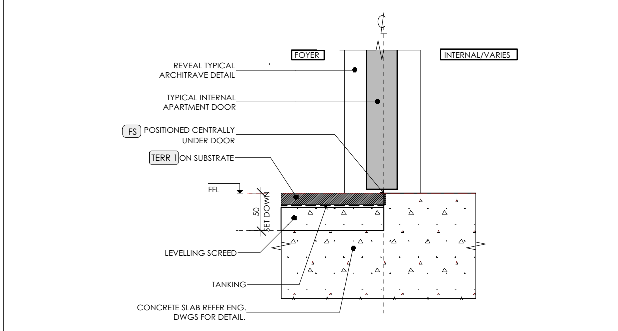
D FOYER THRESHOLD Scale: 1:5
